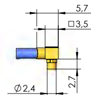
MMPX™-m (angular 90°)
